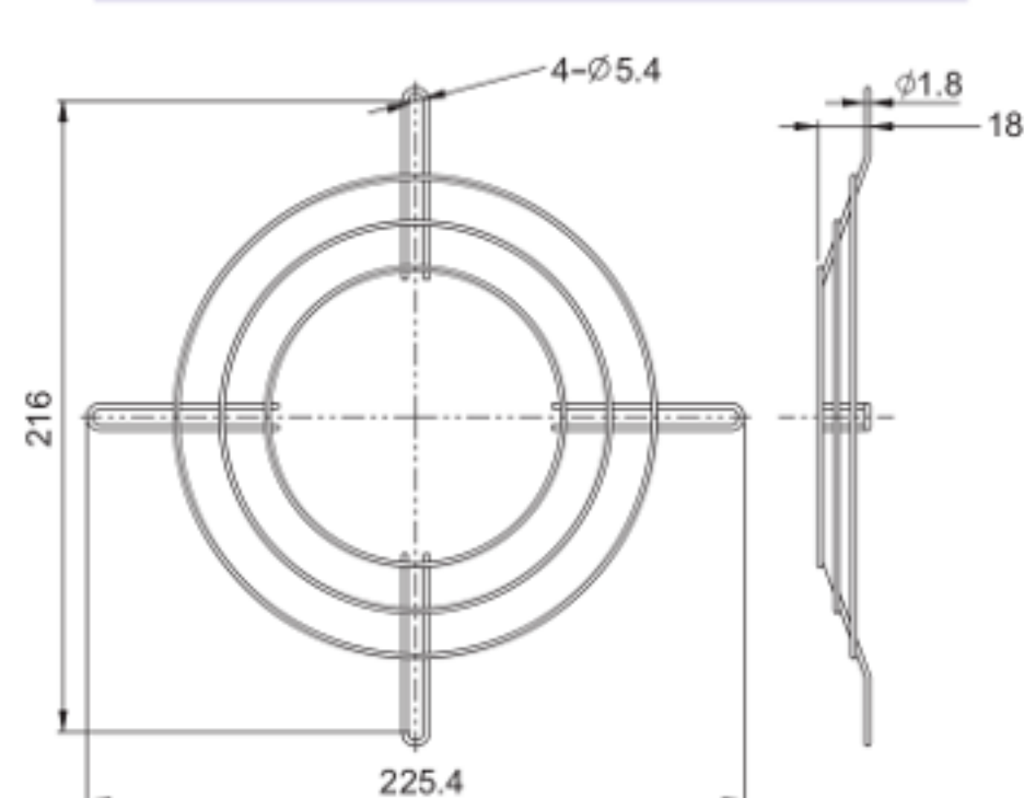
FG-18B For 176mm Fan
