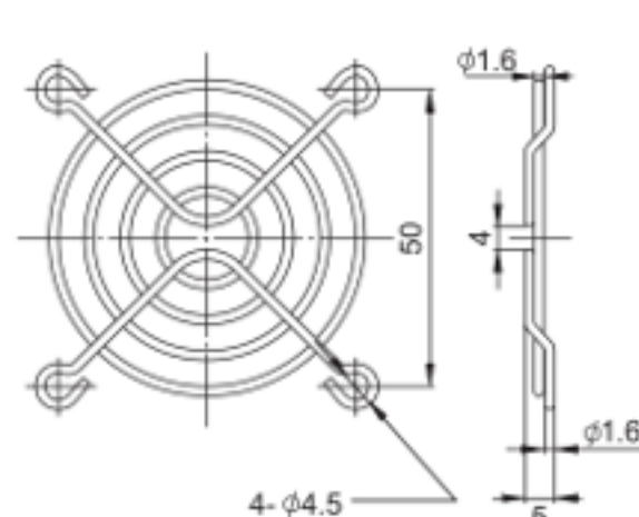
FG-06 For 60mm Fan
