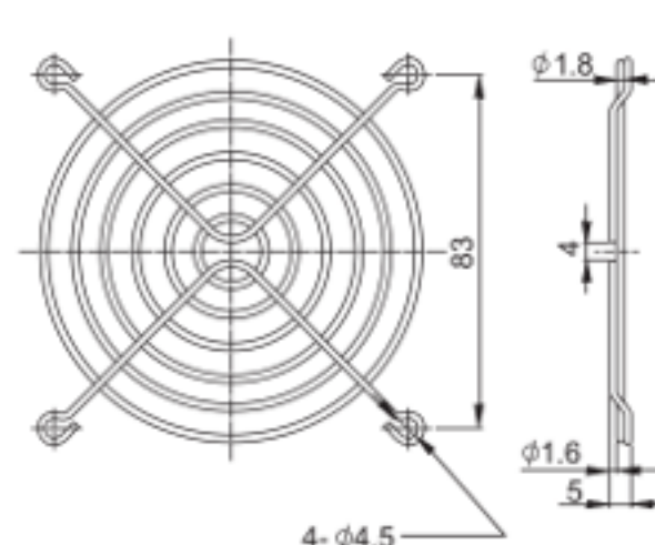
FG-09 For 92mm Fan
