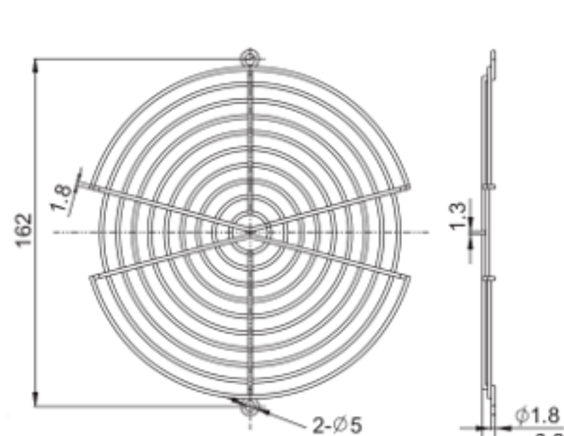
FG-17B For 172mm Fan
