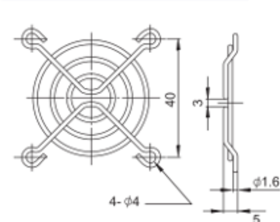
FG-05 For 50mm Fan
