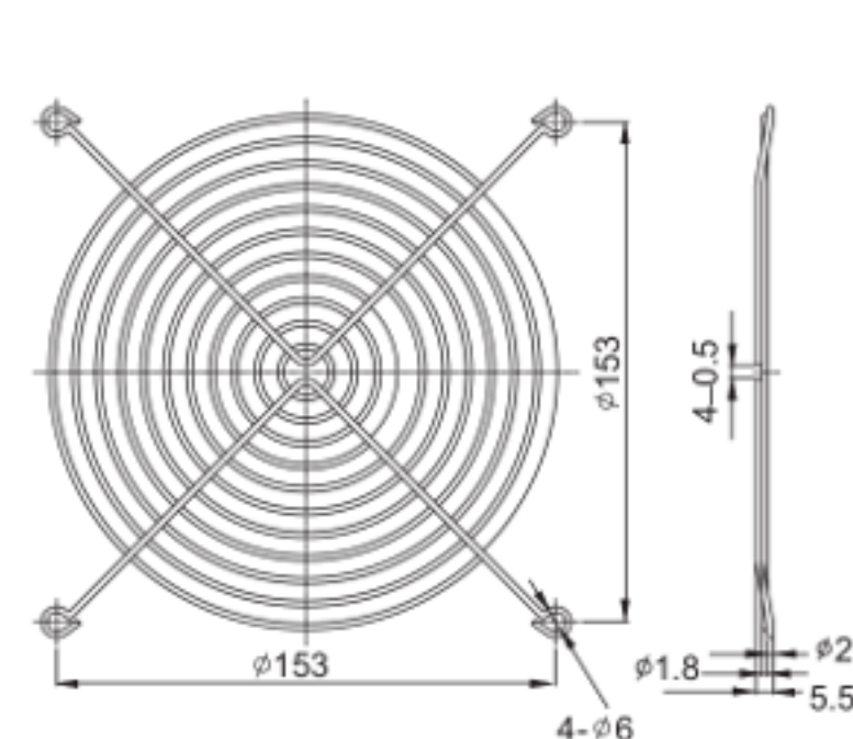
FG-18A For 176mm Fan
