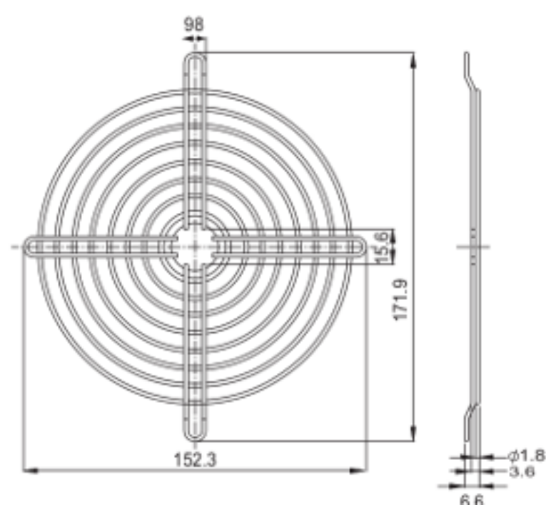
FG-18B For 176mm Fan
