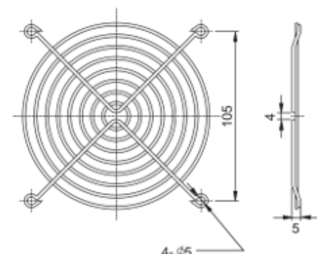
FG-12 For 120mm Fan
